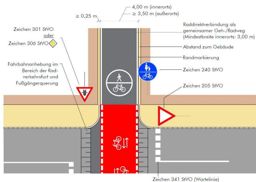
Abbildung 64: Musterblatt RDV-3: Selbstständige Führung (gemeinsamer Geh-/Radweg) außerorts 120
