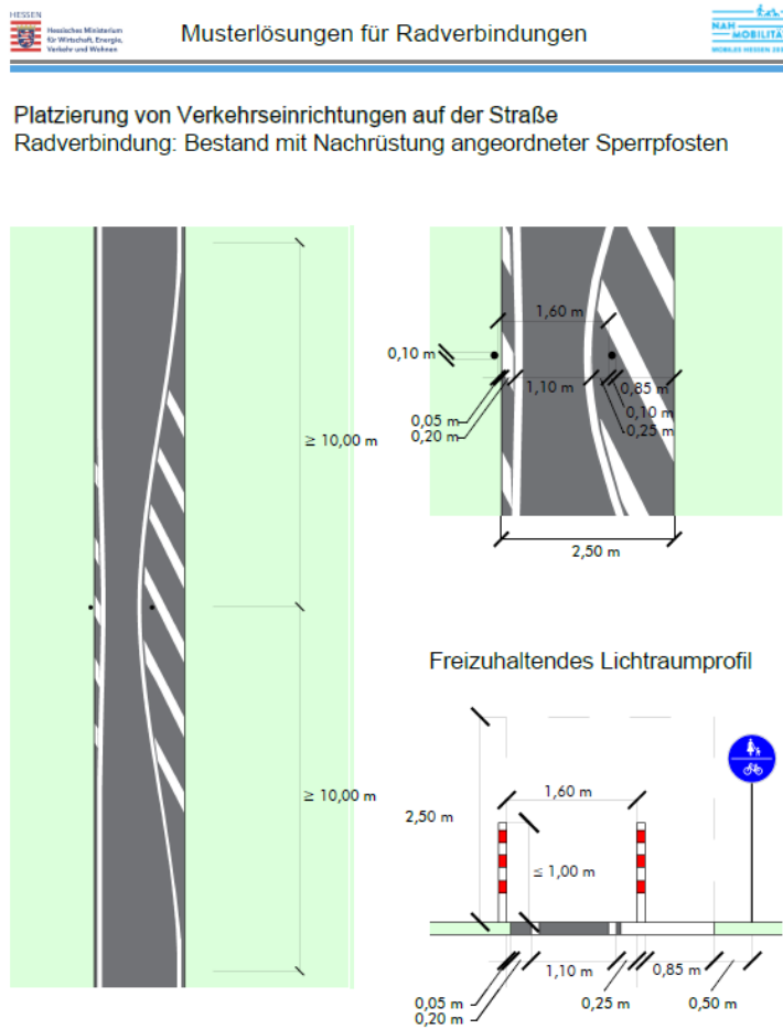
Abbildung 77: Musterlösung Poller 141
