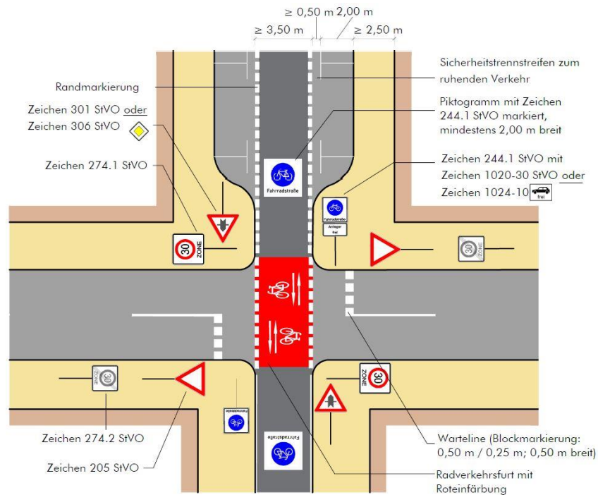
Abbildung 66: Musterlösung RDV-12: Führung einer Fahrradstraße innerorts 122
