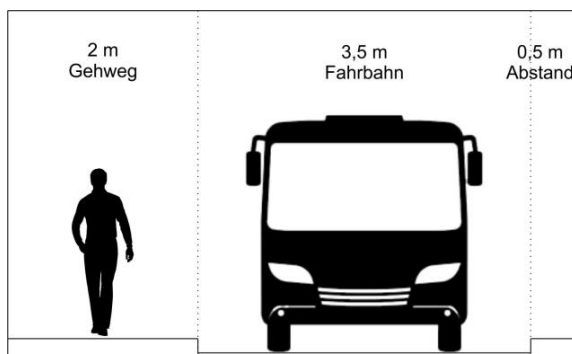
Abbildung 70: Mögliche Aufteilung in der Unterführung Niester Straße
