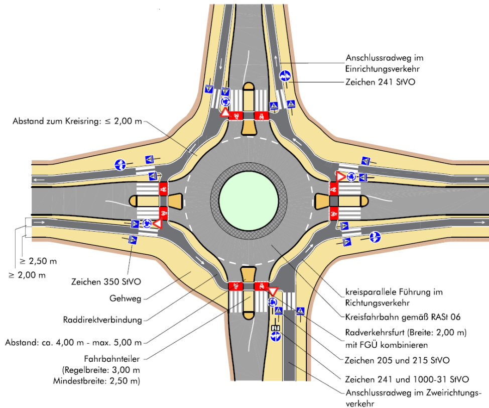
Abbildung 67: Bevorrechtigte Führung auf umlaufenden Radwegen im Kreisverkehr 124
