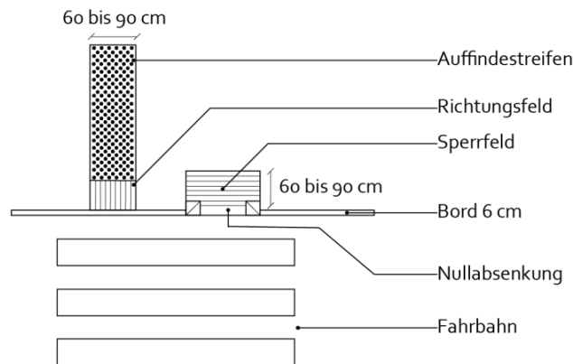
Abbildung 4: Gestaltung von barrierefreien Querungen 10
